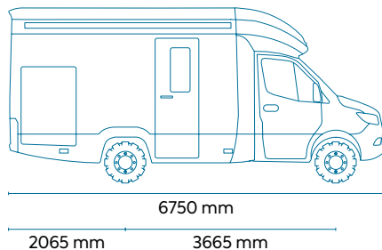
Monoscocca in fibra di carbonio
